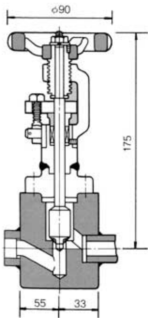
NKGDレンバルブ DV15
