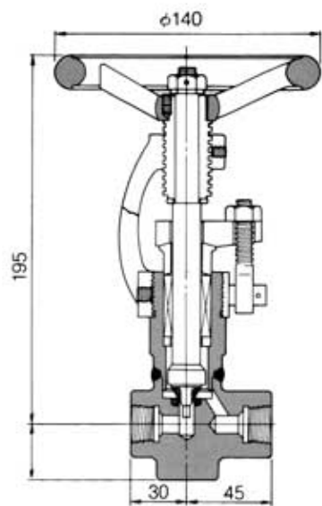
NKGDレンバルブ DV18
