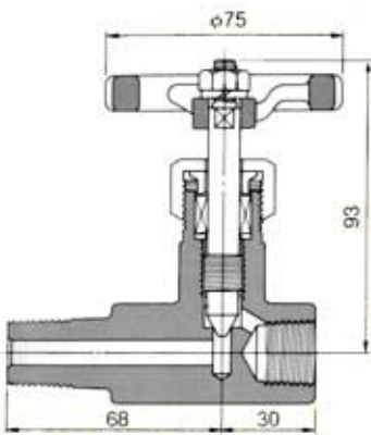
NKGDレンバルブ DV21
