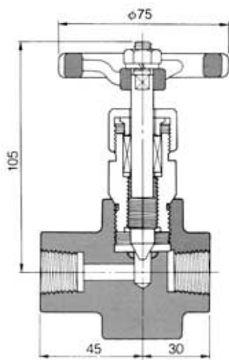
NKGDレンバルブ DV25
