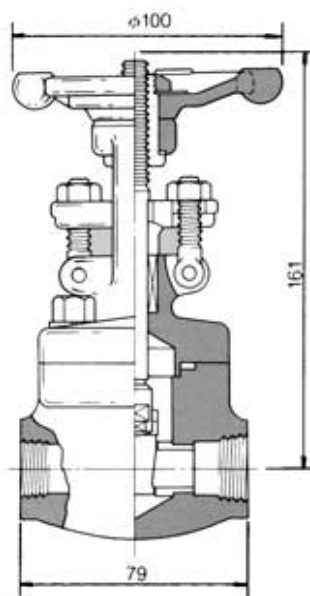
NKGドレンバルブ DV51
