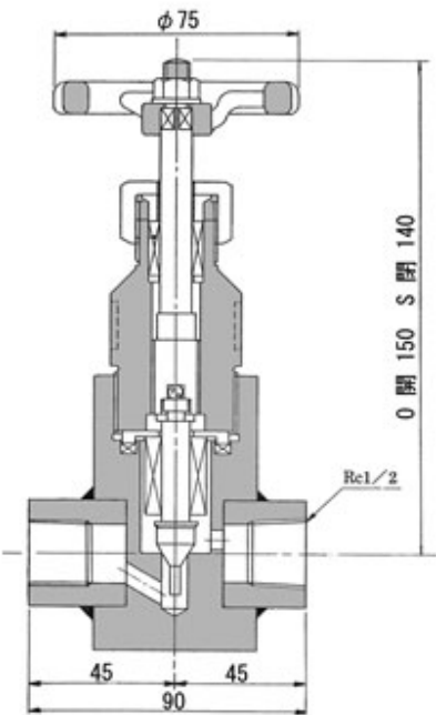
NKGDレンバルブ DV61
