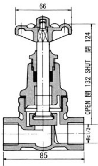
NKGDレンバルブ DV65
