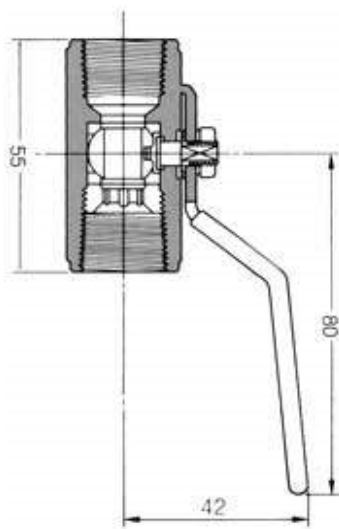
NKGドレンバルブ DV70
